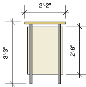
KIOSK COUNTER
