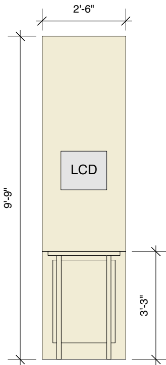
KIOSK
